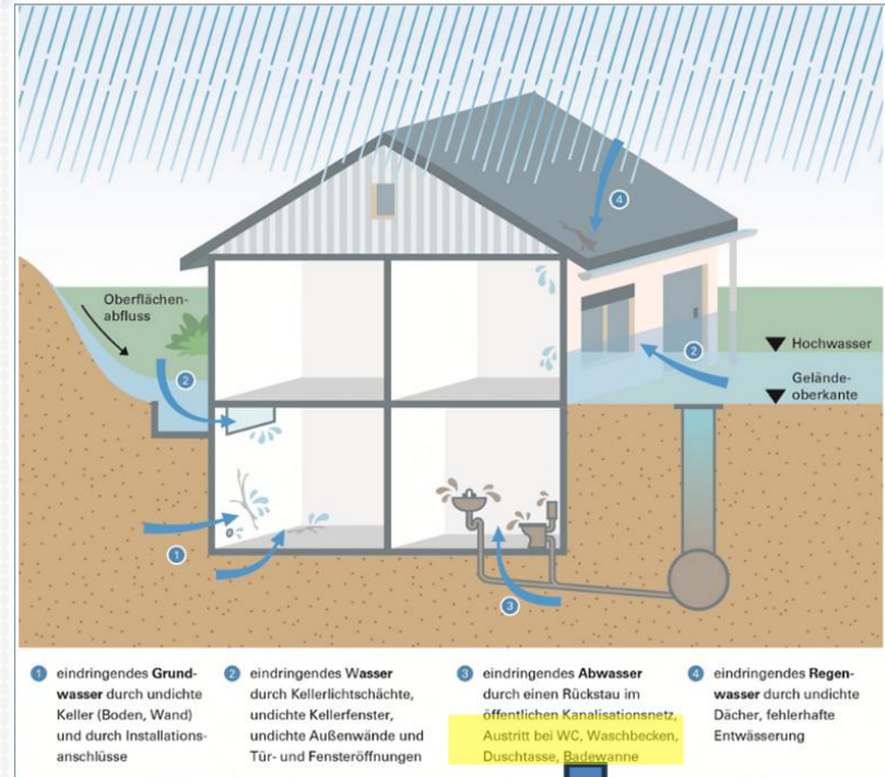
Abb. 4: Mögliche Wege über die Wasser in ein Gebäude eindringen kann
