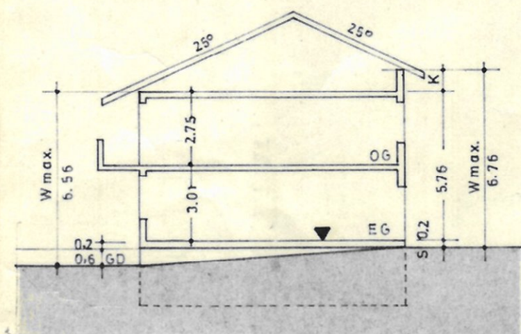
E E+O+S AUSNAHMSWEISE SOCKEL BIS 60cm ALS GELÄNDAUSGLEICH ZUGELASSEN. ALTERNATIVE: VG WIE SCHEMA „G“, EINSEITIGER KNIESTOCK VORGESCHR.
