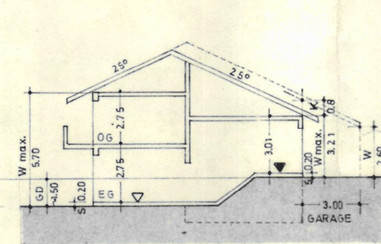
G E+1/2O+VG BEI GARAGENANBAU EINSEITIGER KNIESTOCK ZUGELASSEN.
