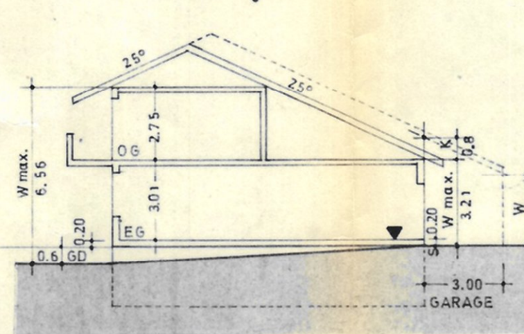
F E+1/2O+S AUSNAHMSWEISE SOCKEL BIS 60cm ALS GELÄNDAUSGLEICH ZUGELASSEN. ALTERNATIVE: VG WIE SCHEMA „G“, BEI GARAGENANBAU EINSEITIGER KNIESTOCK ZUGELASSEN.
