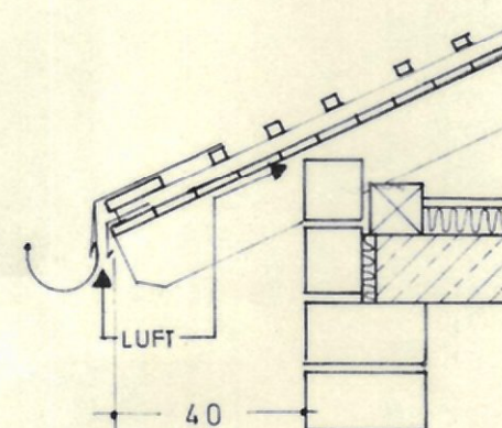
MINDESTDACHÜBERSTAND AN DER TRAUFE
